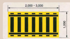
踏切マット(片面)
